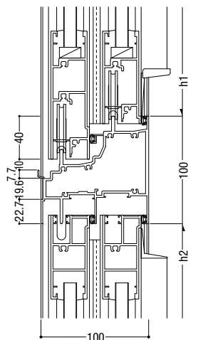
5 インベイ外倒し排煙 / 外動片引き
