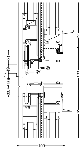
8 インベイ外倒し排煙 / 両袖可動
