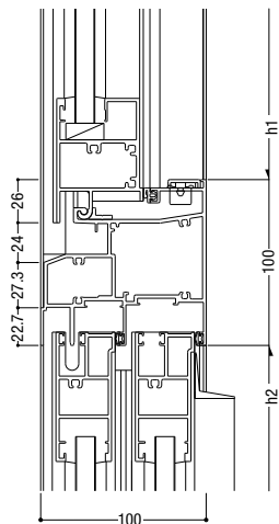
6 FIX / 外動片引き
