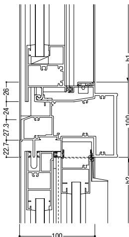
12 引違い / FIX
